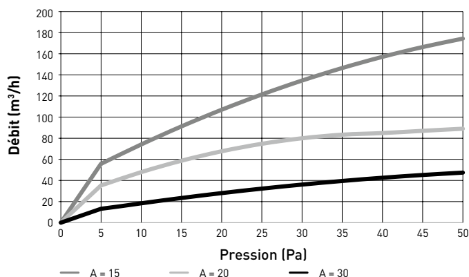
Courbe de pression / débit DucoVent Basic
